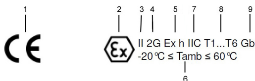
Рис. 10-1 Пример изображения — Маркировка АTEX
